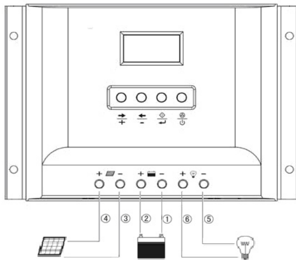
Рис. 1 Последовательность подключения оборудования к контроллеру
