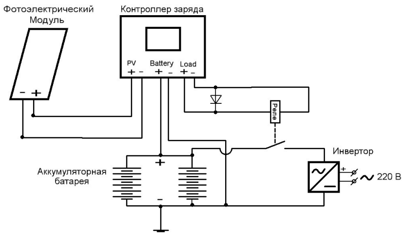
Рис. 2 Схема подключения контроллера и инвертора в системе
