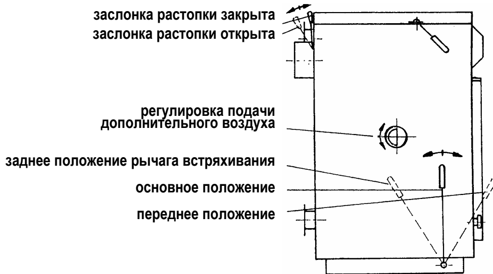
Рис.3 Элементы управления
