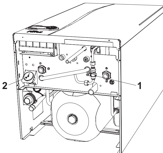
fig. 16 - Rubinetto di caricamento
