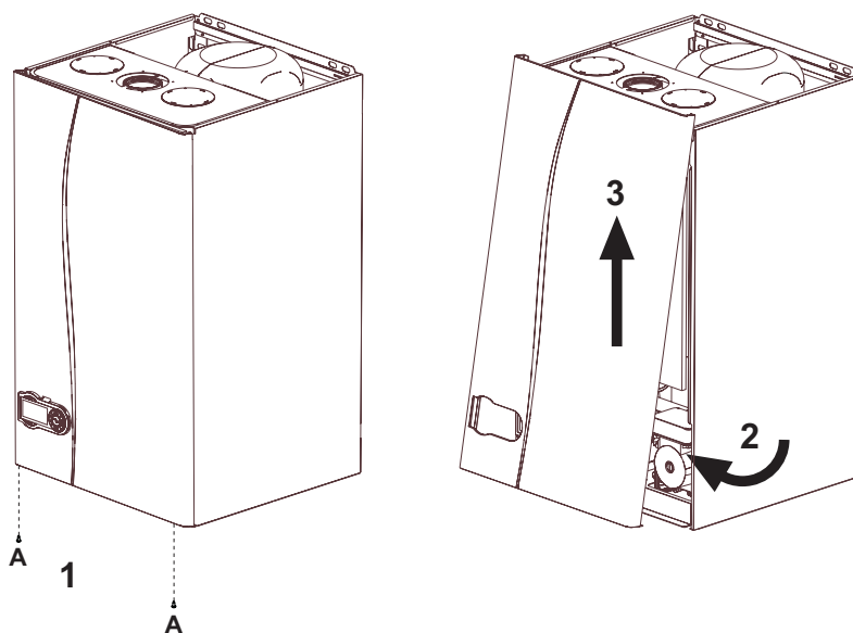
fig. 28 - Apertura mantello
