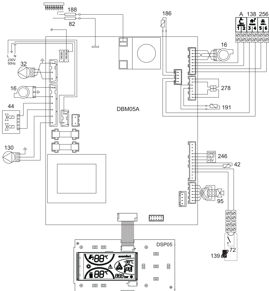
fig. 34 - Schema elettrico
