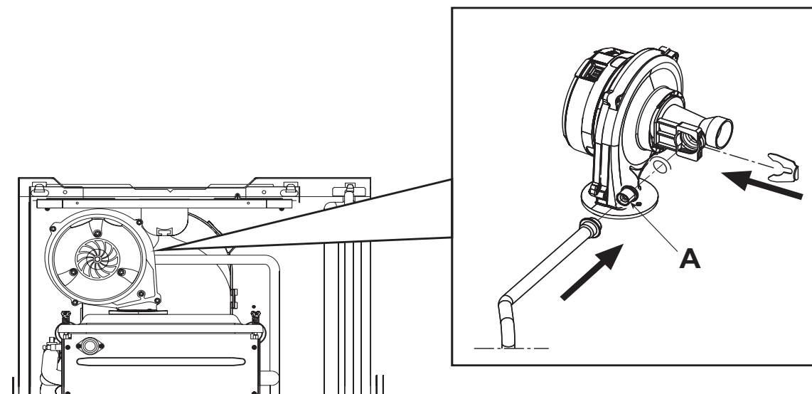
fig. 26 - Sostituzione ugello gas
