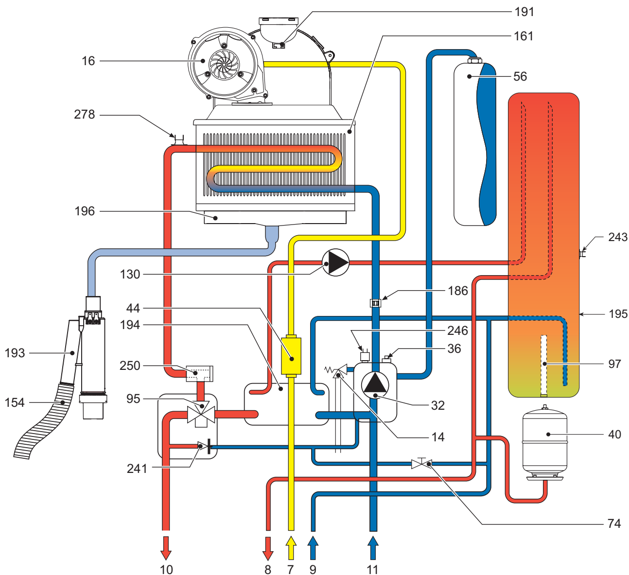
fig. 32 - Circuito idraulico
