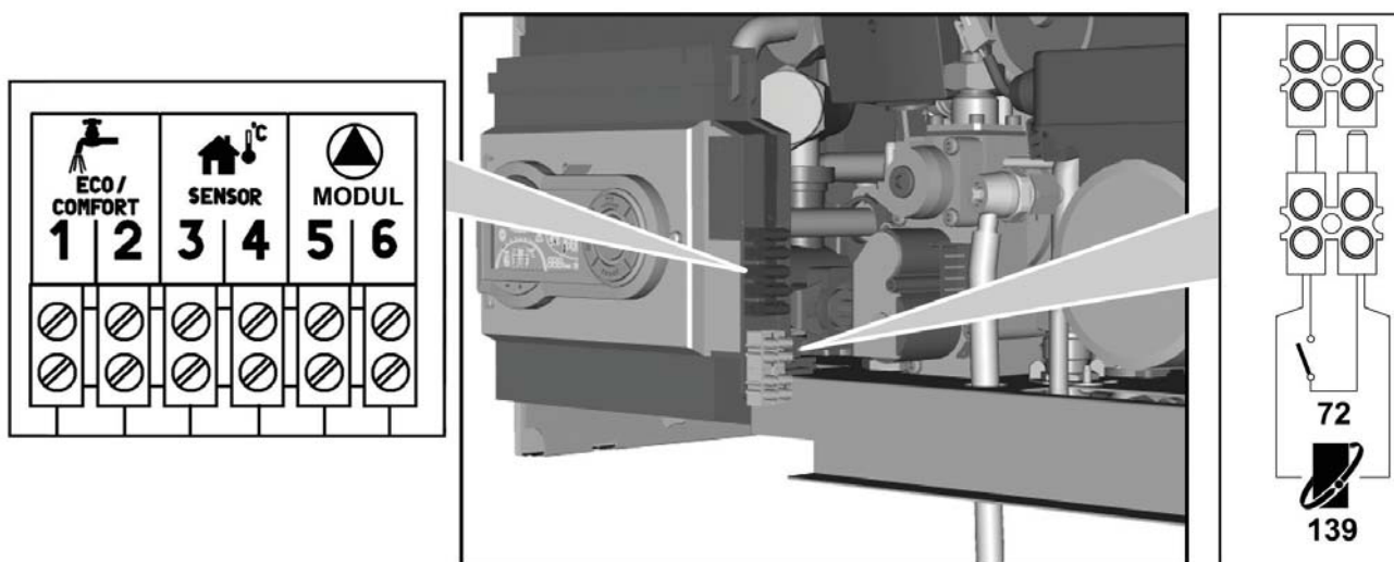
fig. 18 - Accesso alla morsettiera
