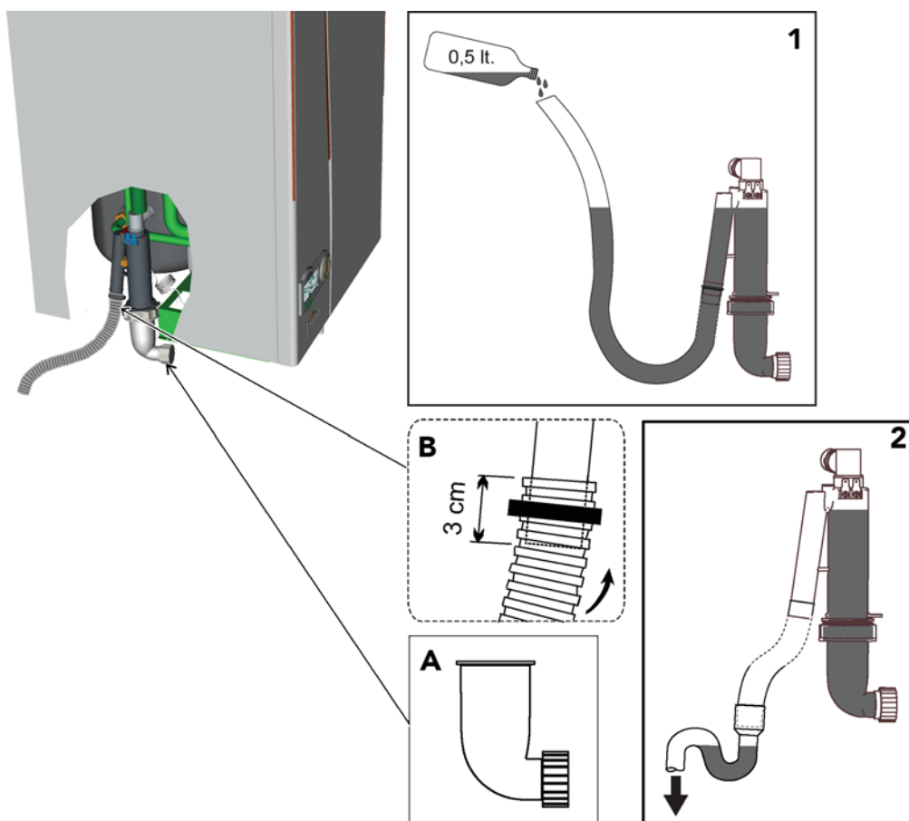
fig. 25 - Scarico condensa
