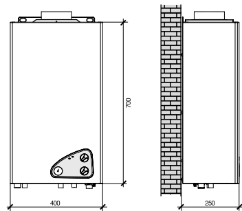
Vela Compact CTN 24 AF
