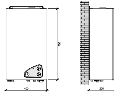
Vela Compact CTFS 24 AF
