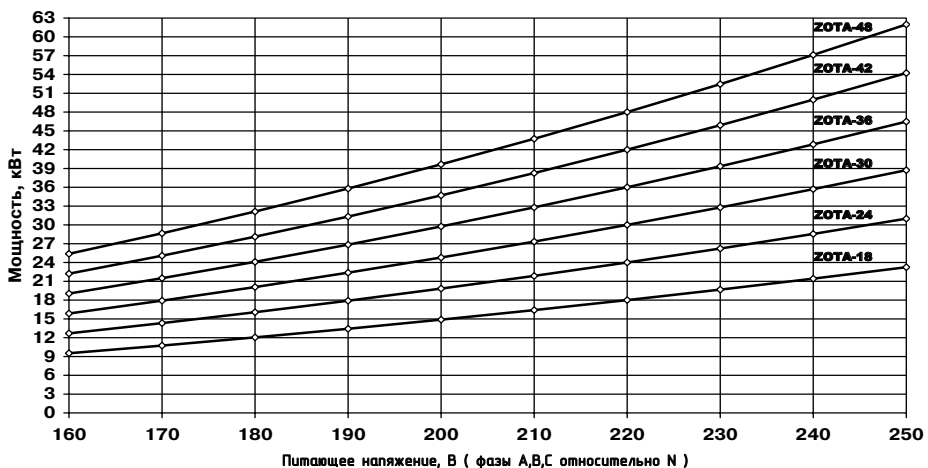
Рис.7 График изменения мощности водонагревателя в зависимости от питающего напряжения
