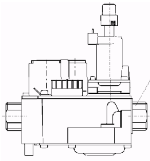
Газовый клапан Газовая диафрагма Прокладка
